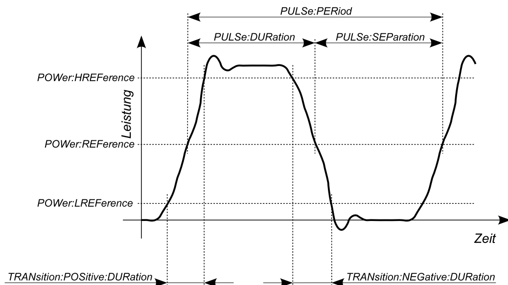
Bild 6-8 Zeitparameter und Referenzpegel eines Traces
